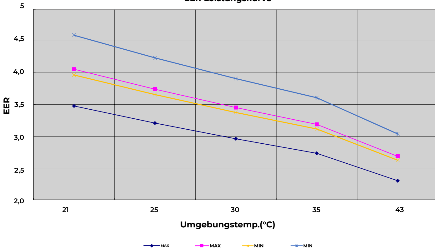
EER Leistungskurve
