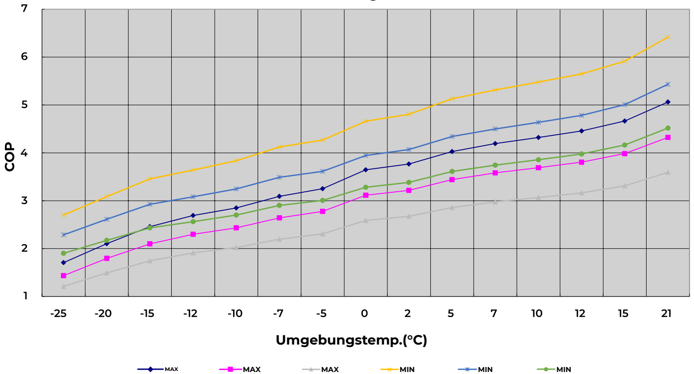
COP Leistungskurve
