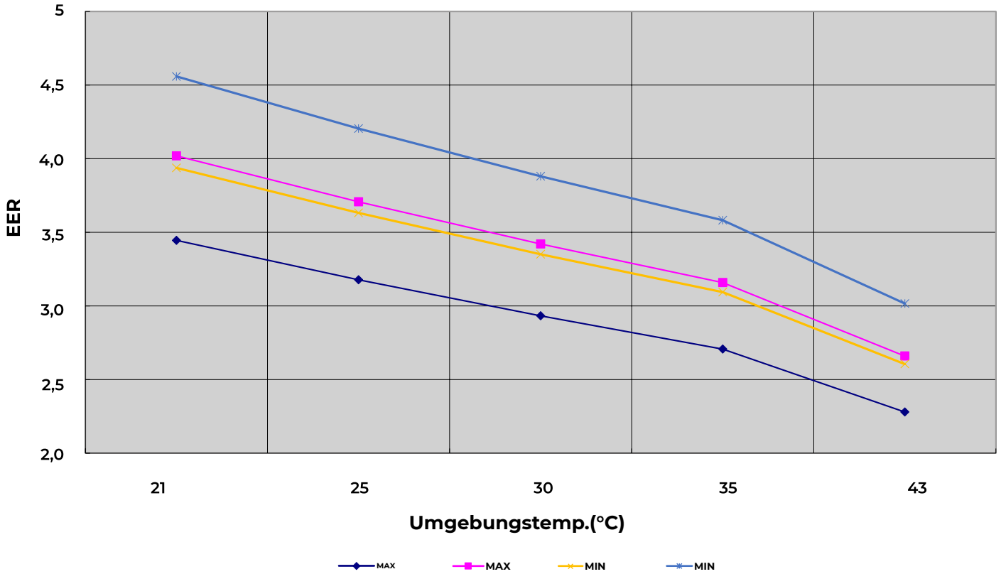
EER Leistungskurve
