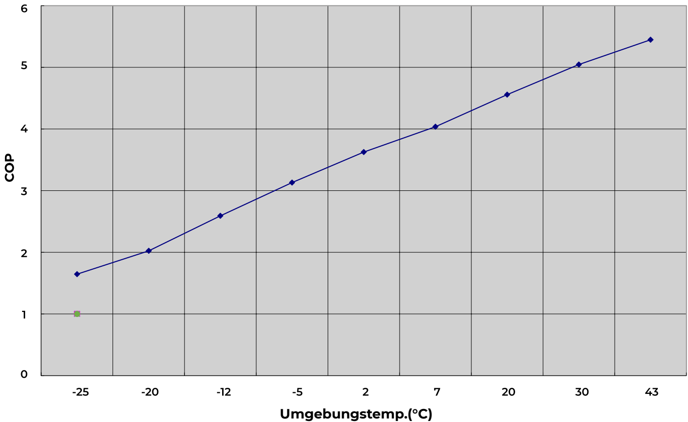
COP Leistungskurve
