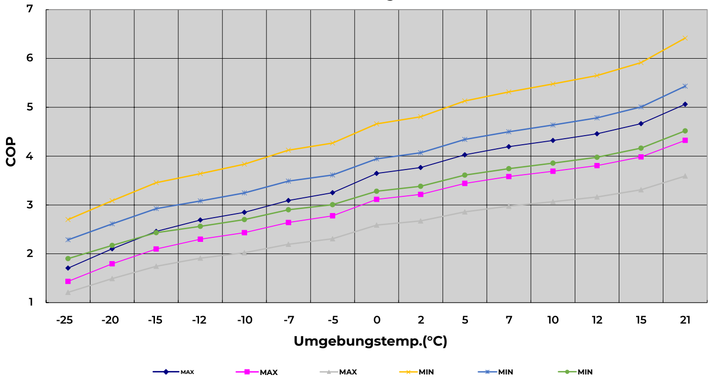
COP Leistungskurve
