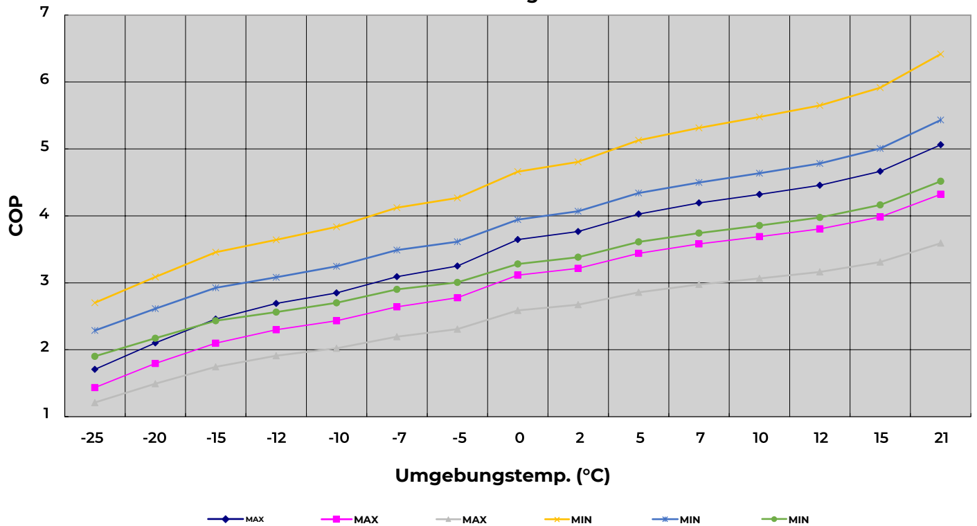
COP Leistungskurve
